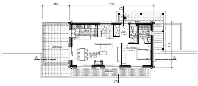
PLAN DU REZ SUPÉRIEUR
