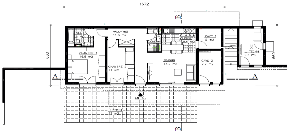
PLAN DU REZ INFÉRIEUR
