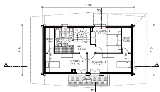
PLAN DES COMBLES
